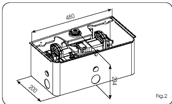
3.1. Standardná verzia obr.2
