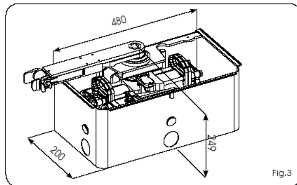
3.2. Verzia s unášecou pákou a mech.odblokovaním obr.3
